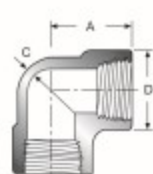
90° 弯头 90° Elbow
